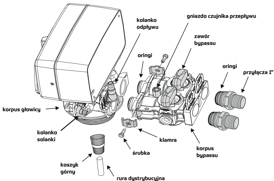
rys.3. Podłączenie bypass
