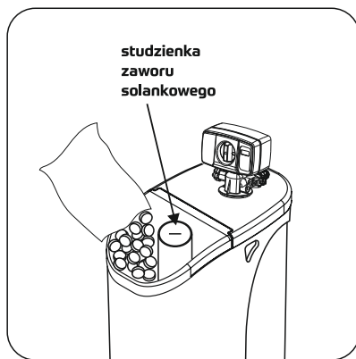
rys. 8. Uzupełnianie soli w urządzeniu kompaktowym
