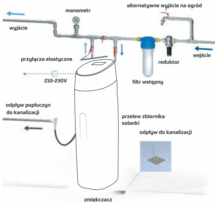
rys.1. Schemat podłączenia zmiękczacza
